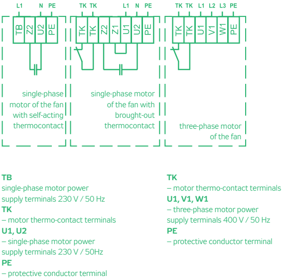
FIGURE 5 – RF FAN WIRING DIAGRAM
